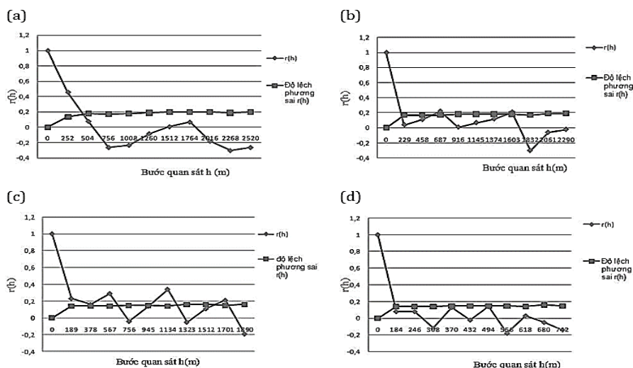
Hình 4. Đồ thị biểu diễn mối quan hệ giữa hàm tương qua định mức r(h) với bước quan sát (h) các vỉa than. a) Vỉa 8V; b) Vỉa 8T; c) Vỉa 9V; d) Vỉa 9T.
